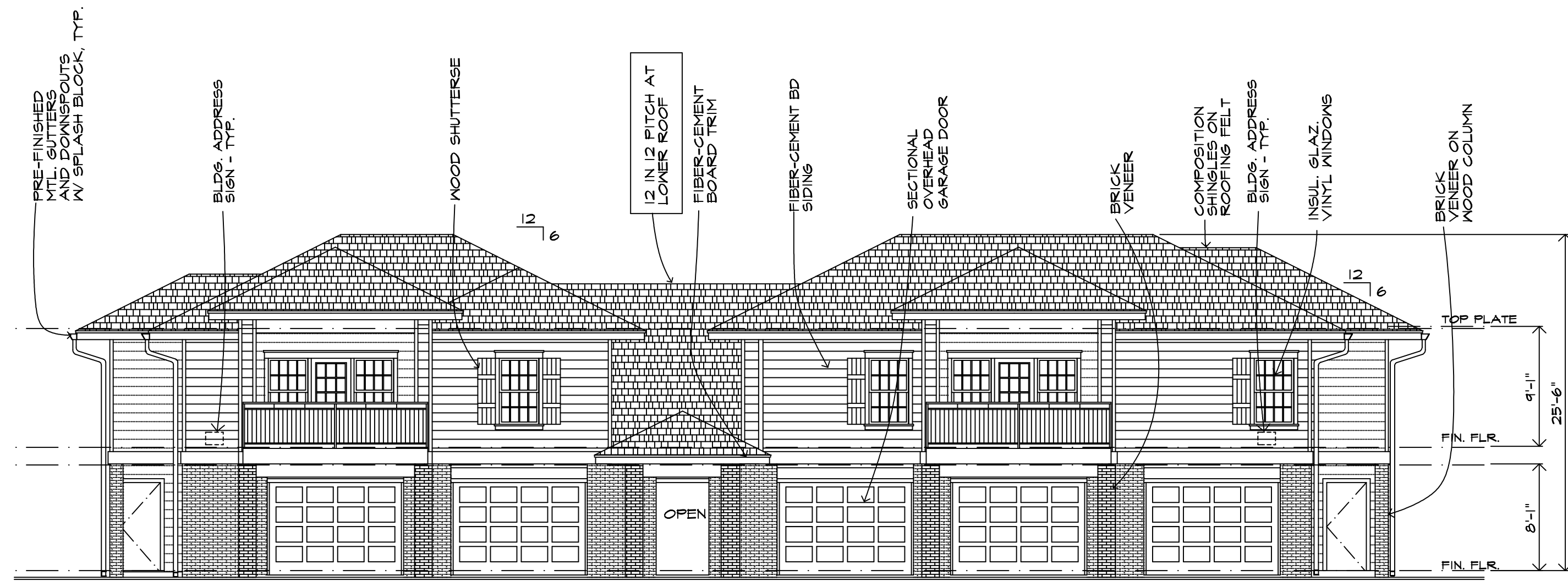
A FRONT ELEV. - A3/B3 1/8"=1'-0"
